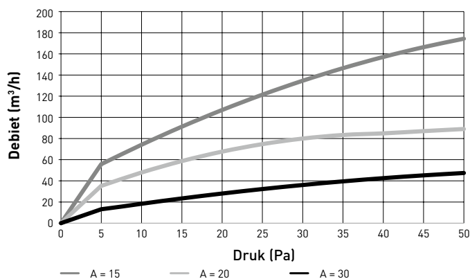
Druk / debiet curve DucoVent Basic
