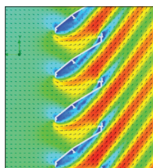
Uitblaas
