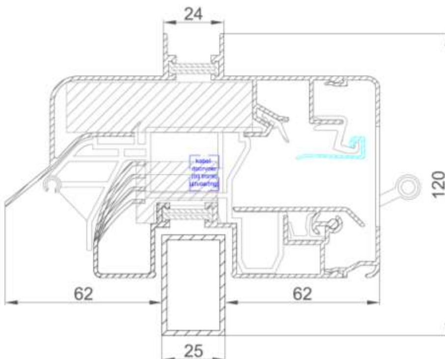
GlasMax 'ZR' – halfplaatsing
