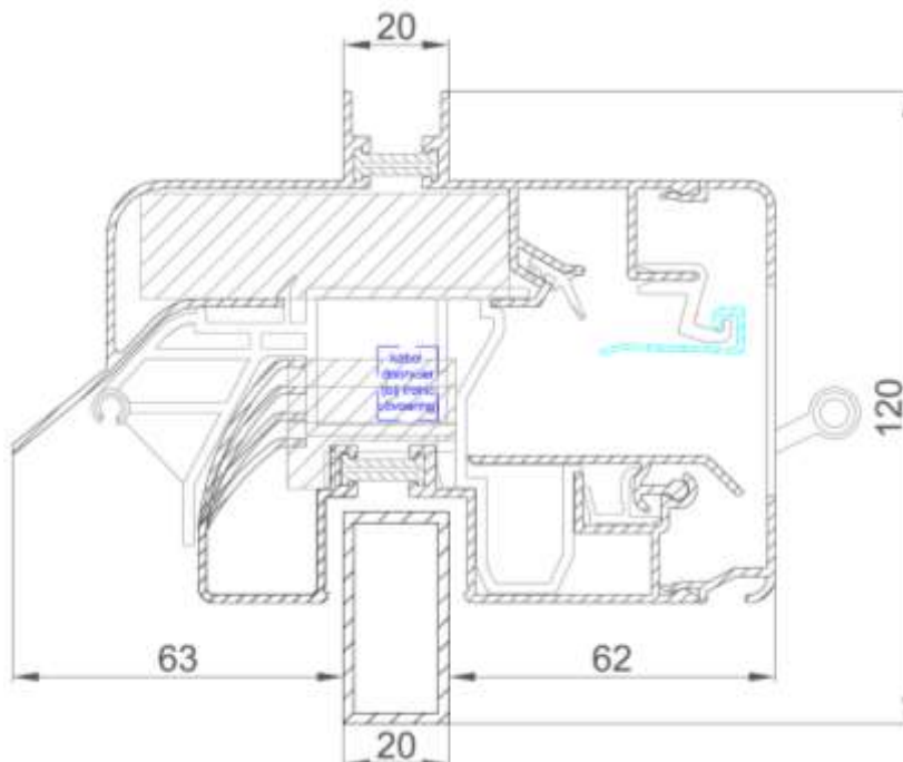
GlasMax 'ZR' – halfplaatsing
