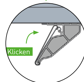
Schiebe-Klick System
