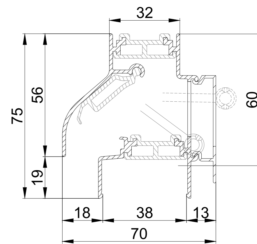
DucoSmart 60 / GG38
