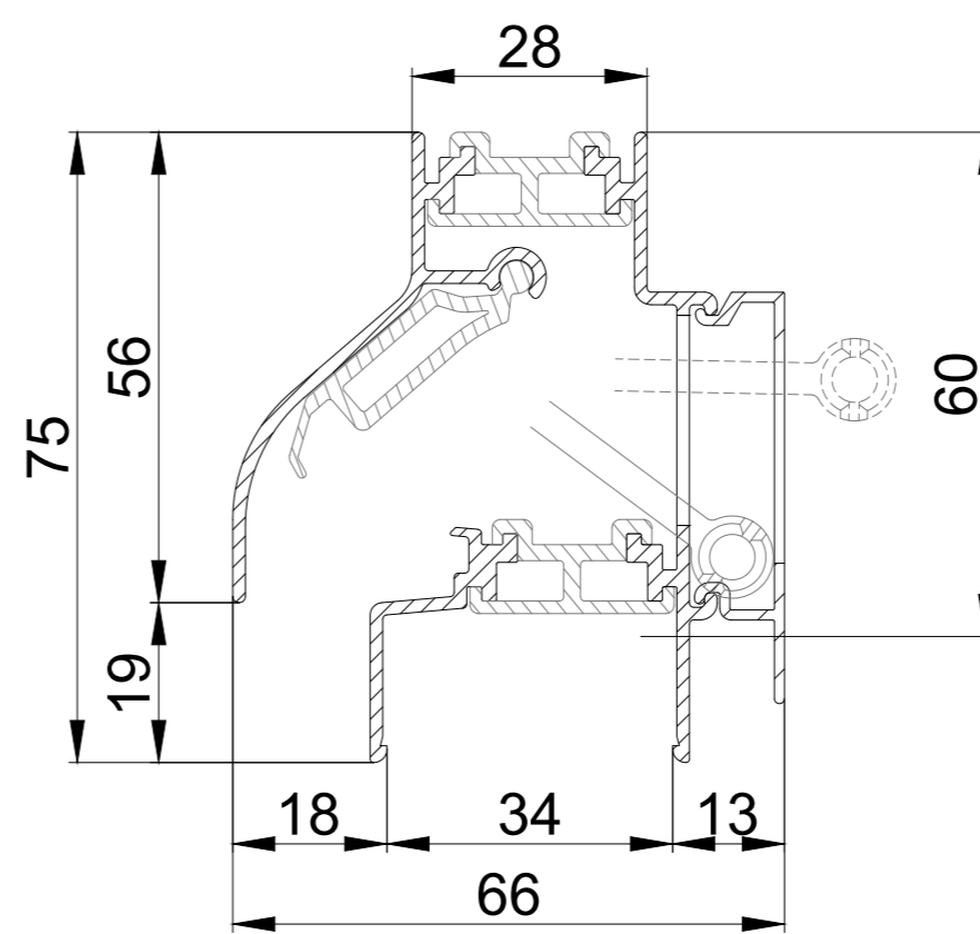
DucoSmart 60 / GG34
