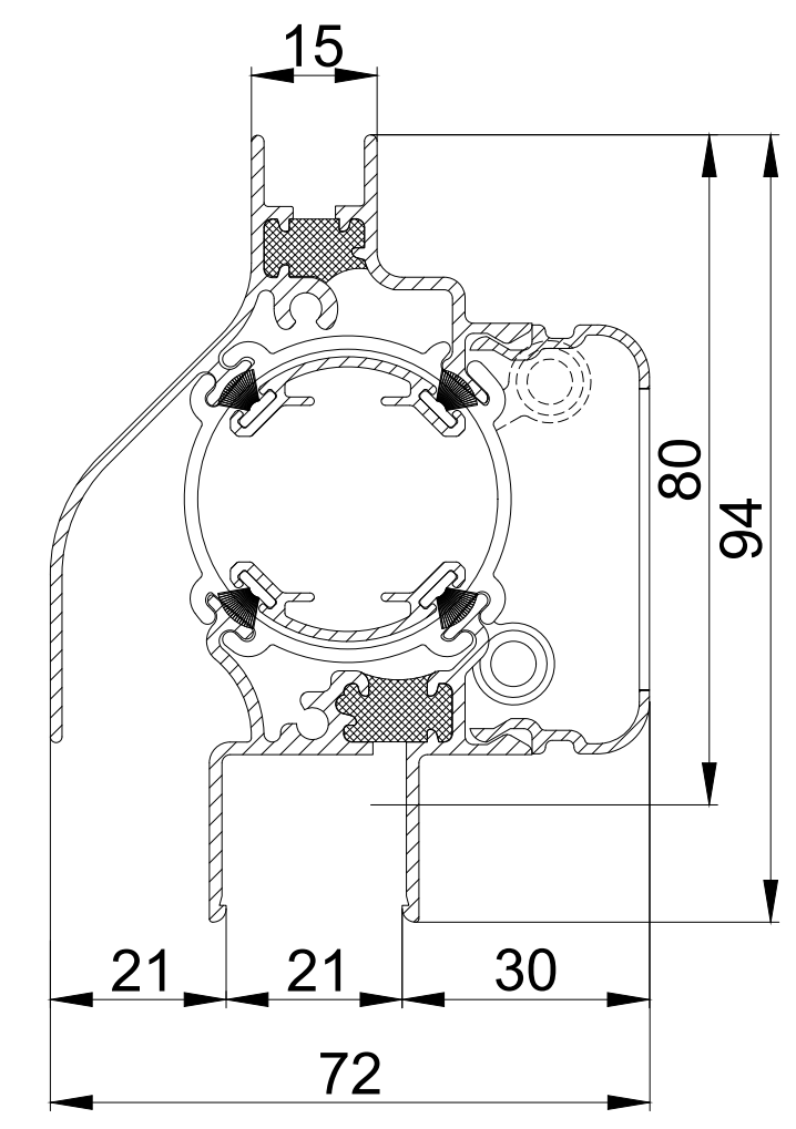
DucoTon 10 / GG21
