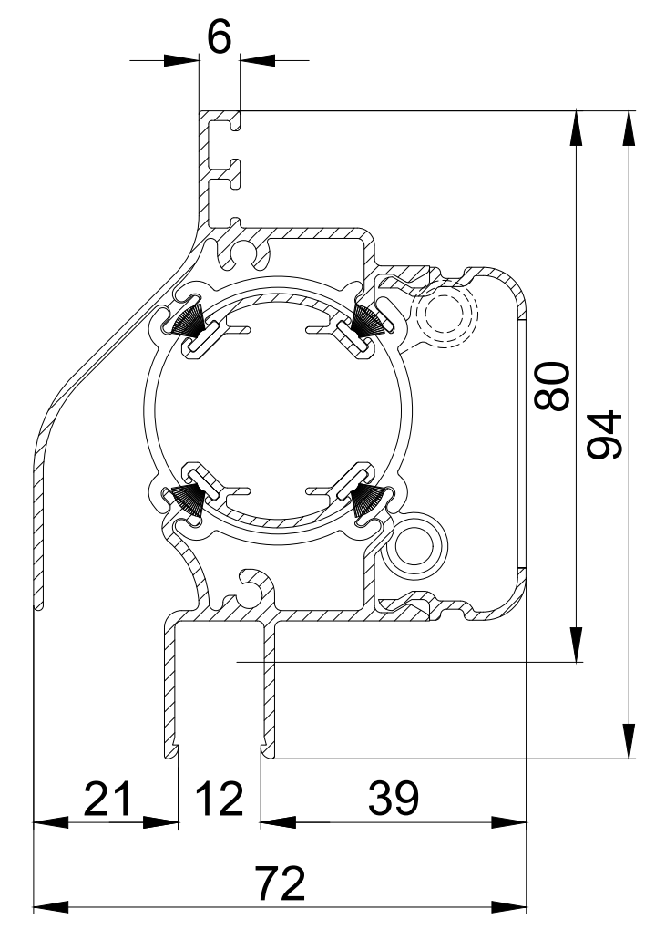
DucoTon 10 / GG12
