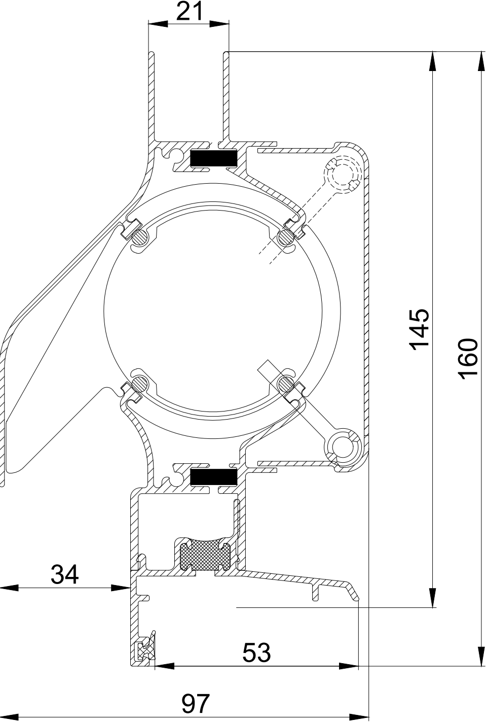
DucoTon 120 / aanslag
