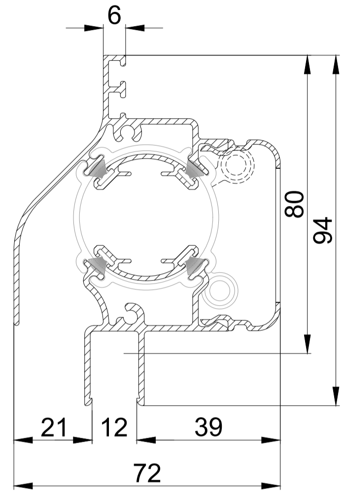
DucoTon 80 / GG12
