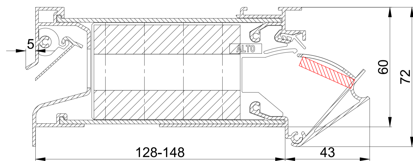
DucoTop 60 ZR Alto
