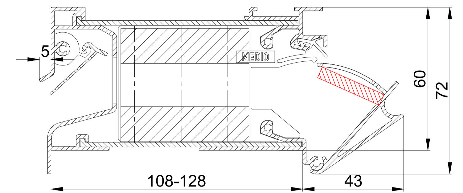
DucoTop 60 ZR Medio
