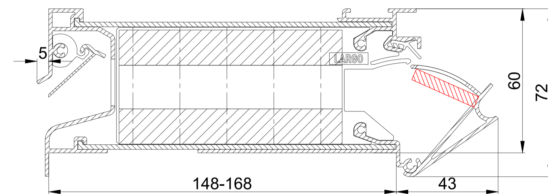
DucoTop 60 ZR Largo
