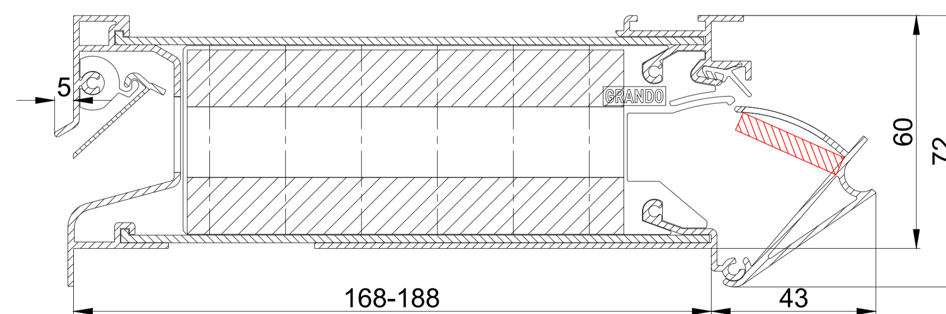
DucoTop 60 ZR Grando
