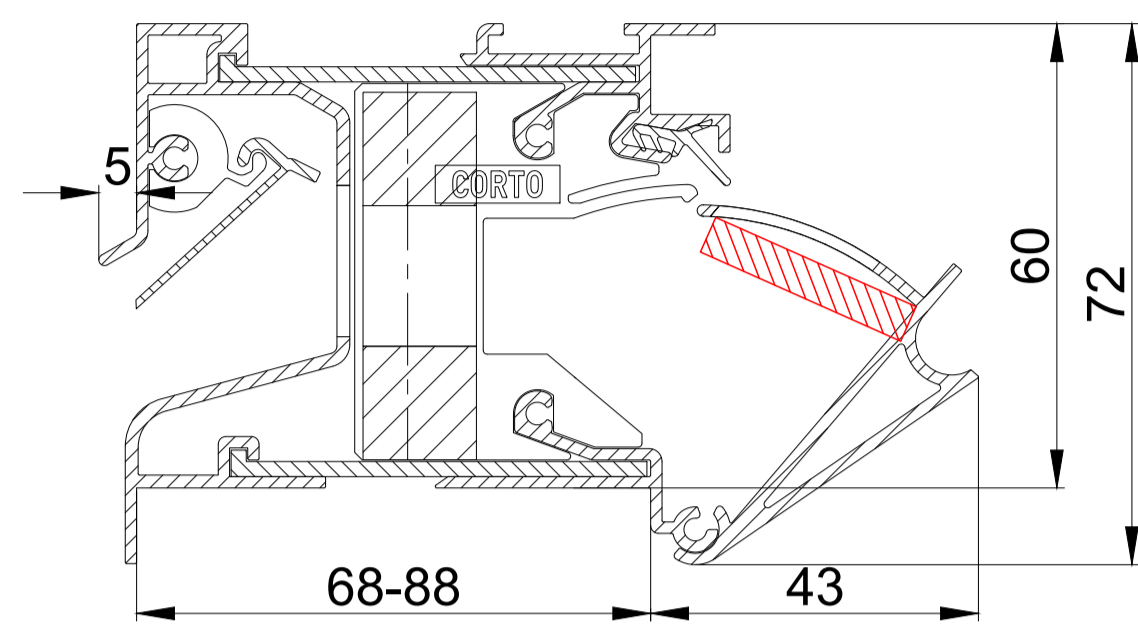
DucoTop 60 ZR Corto
