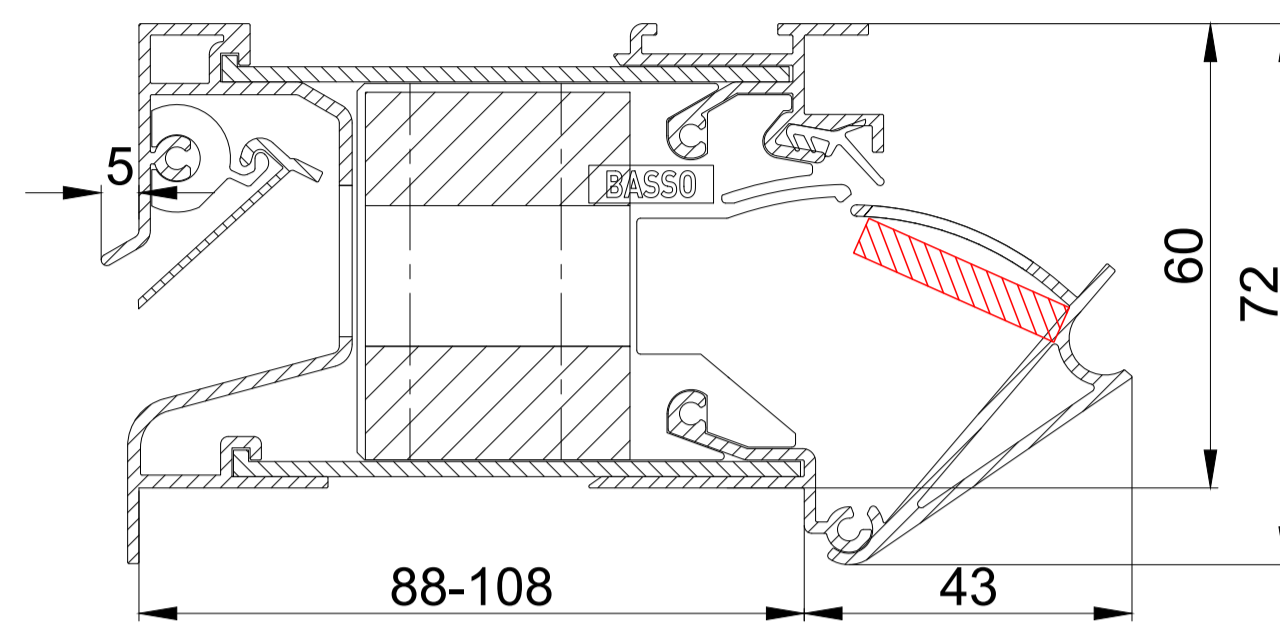
DucoTop 60 ZR Basso
