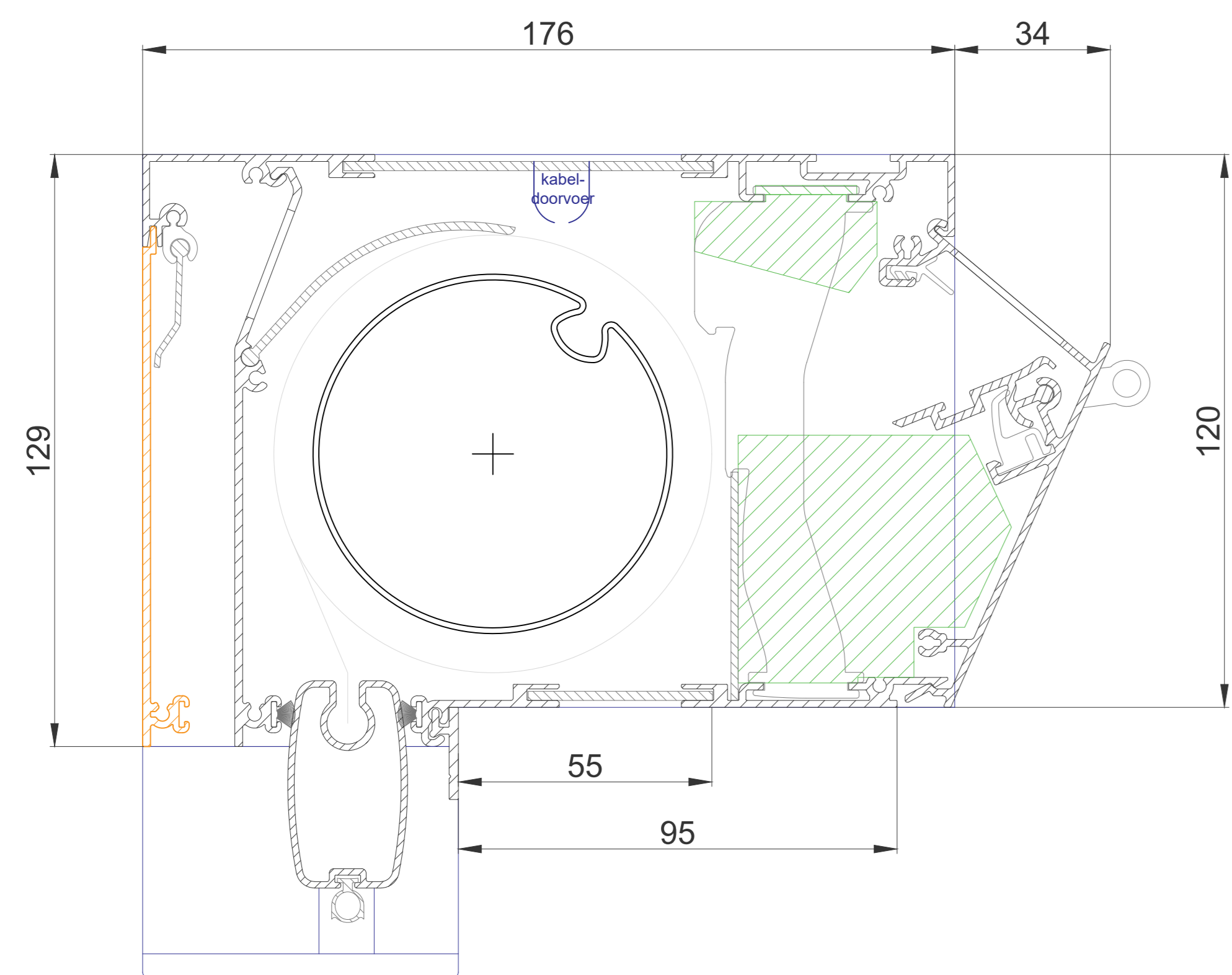
DucoTwin 120 Corto ZR
