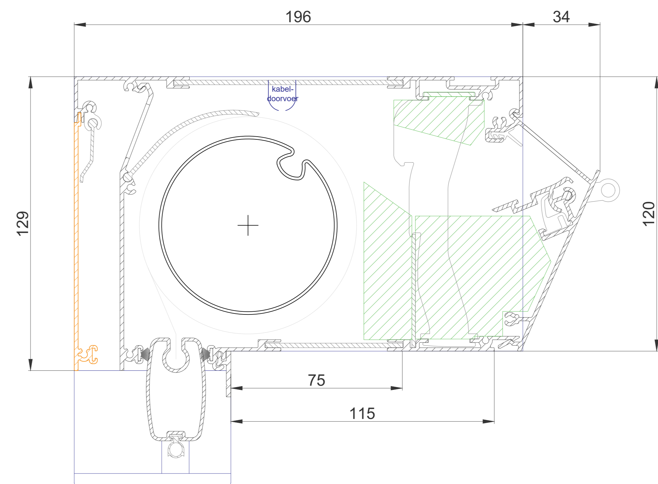
DucoTwin 120 Basso ZR
