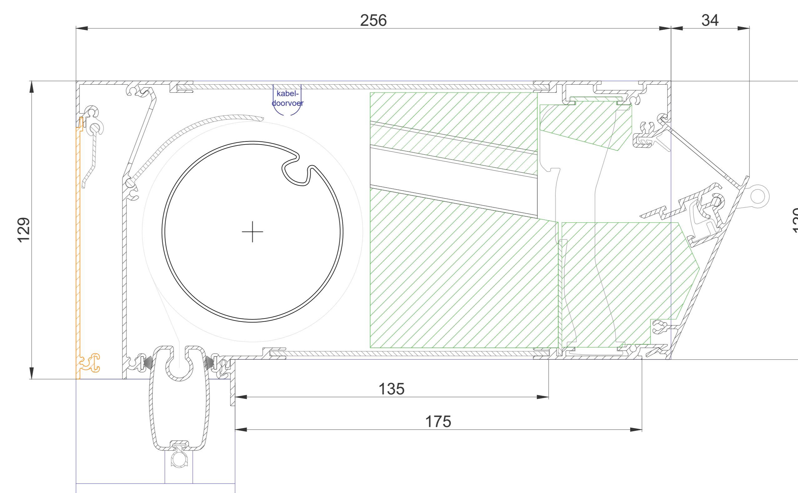
DucoTwin 120 Largo ZR
