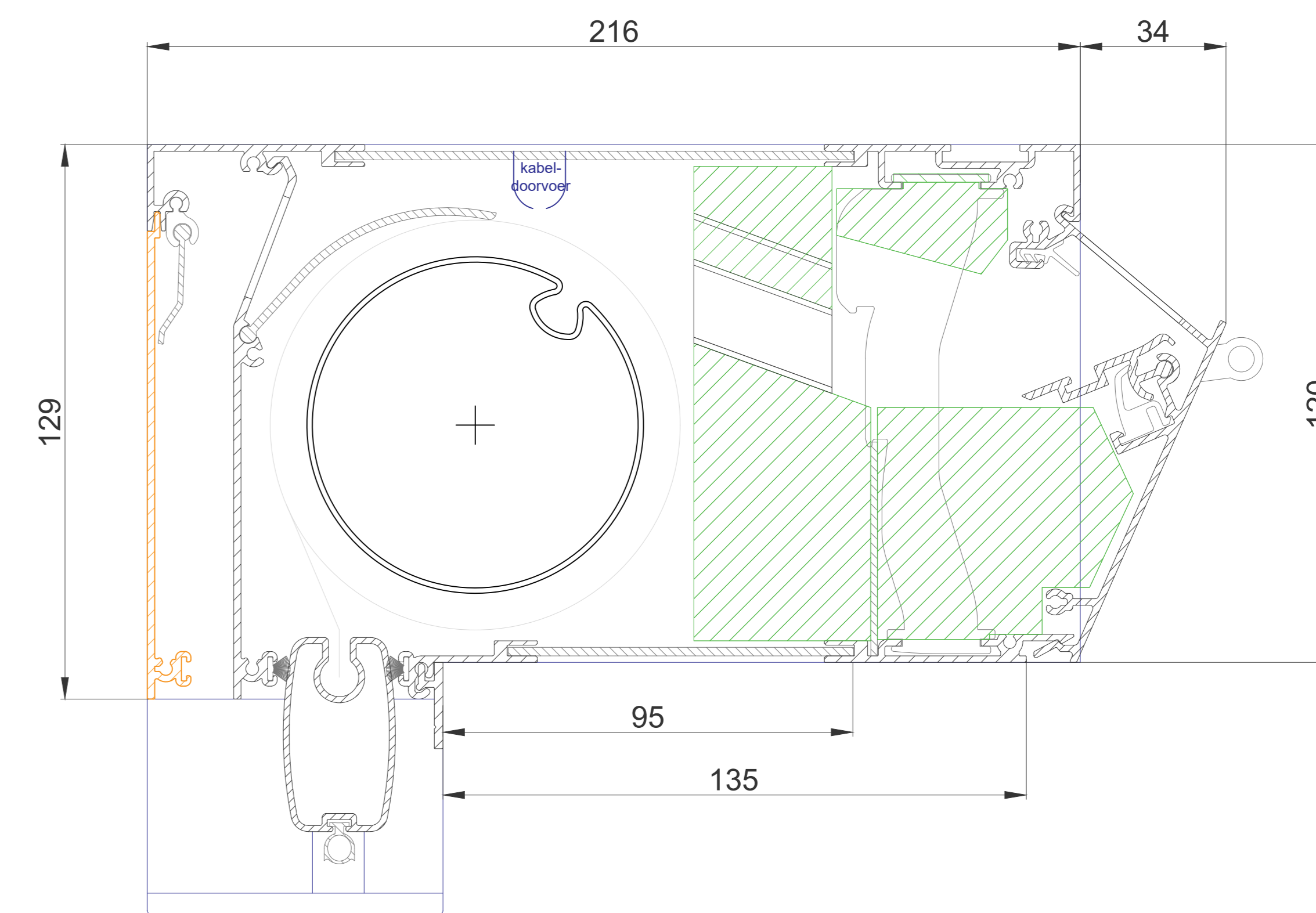
DucoTwin 120 Medio ZR
