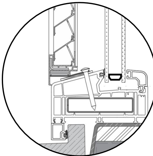
PVC kozijn
