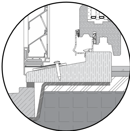
Houten kozijn
