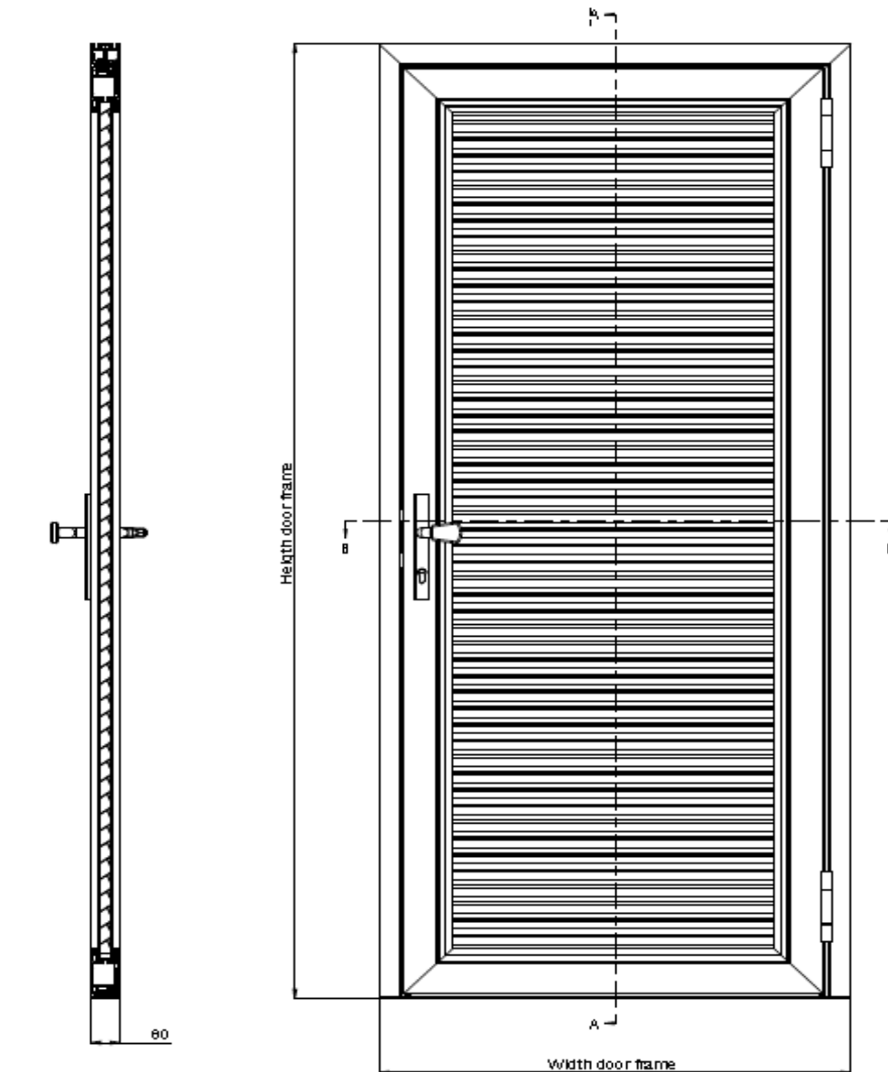
Section A-A
