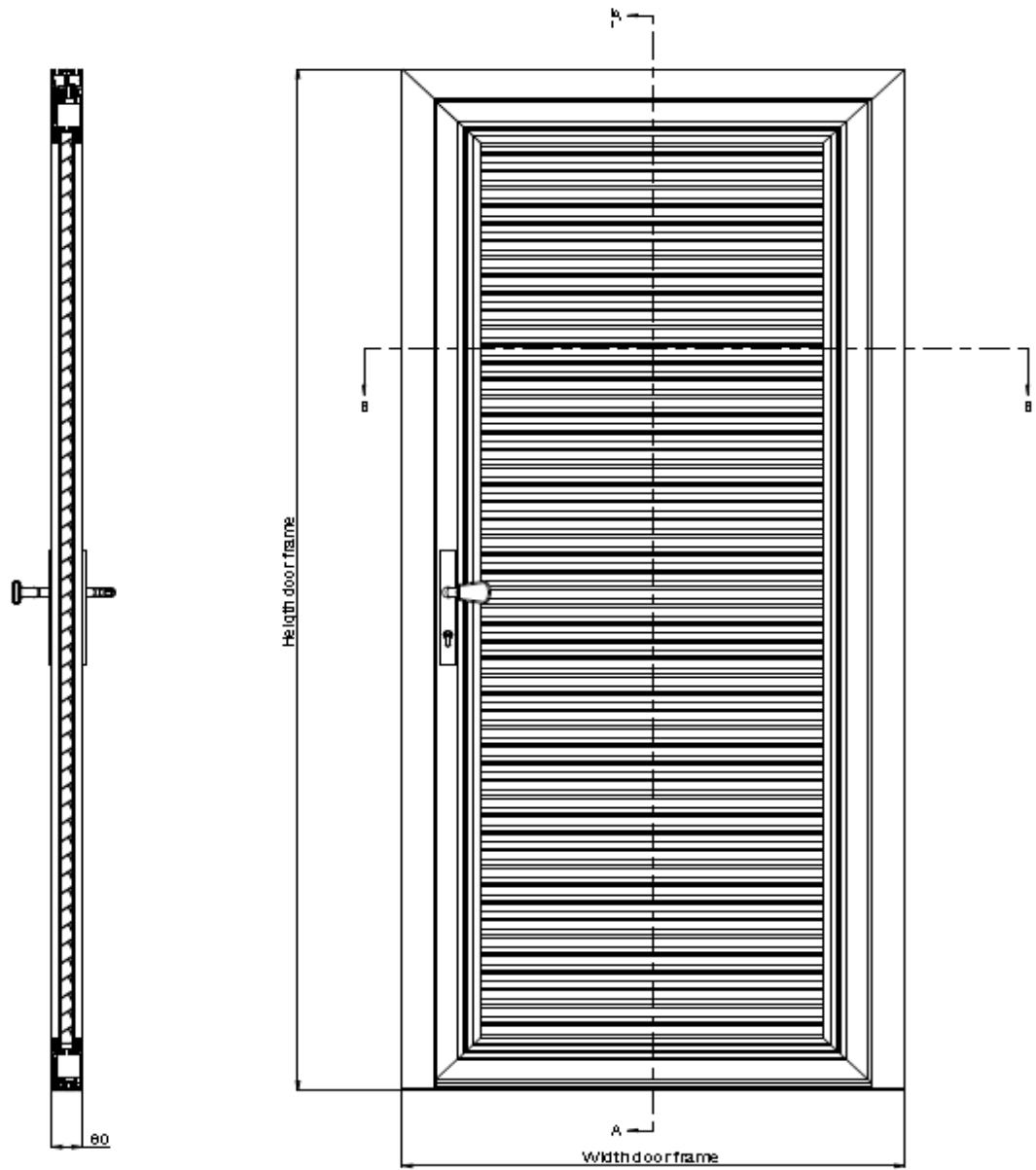
Section A-A
