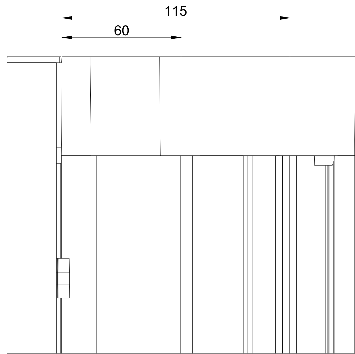
TronicVent Corto
