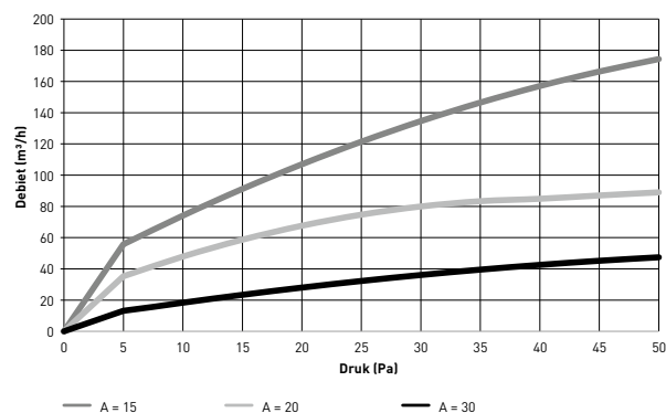
Druk / débit curve DucoVent Basic
