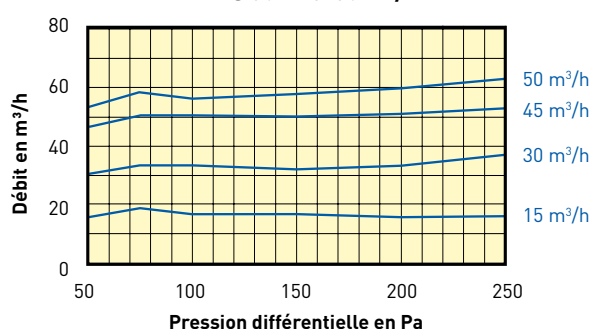
RDR Ø80 - 15-50 m 3 /h
