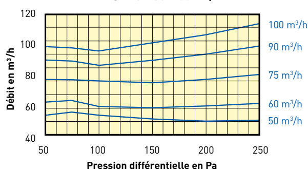
RDR Ø125 - 50-100 m 3 /h
