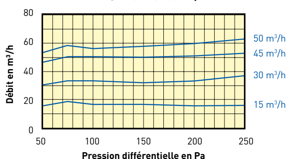
RDR Ø125 - 15-50 m 3 /h
