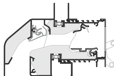
→ GlasVent 16 ZR AK kalfplaatsing
