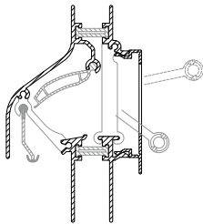
→ DucoKlep 15 'ZR' kalfplaatsing
