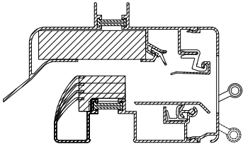
→ GlasMax 'ZR' glasplaatsing
