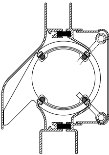
→ DucoTon 18 glasplaatsing
