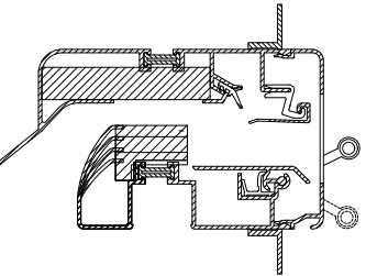
→ GlasMax 'ZR' compacte kalfplaatsing
