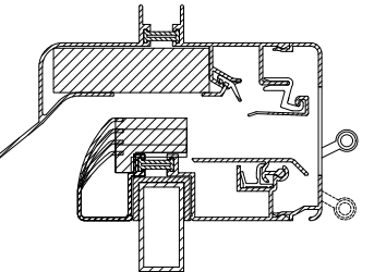
→ GlasMax 'ZR' kalfplaatsing
