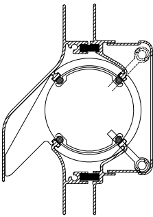
→ DucoTon 18 kalfplaatsing
