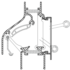
→ DucoKlep 15 'ZR' glasplaatsing
