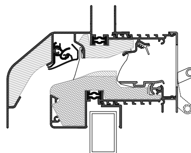
→ GlasVent 16 ZR AK kalfplaatsing
