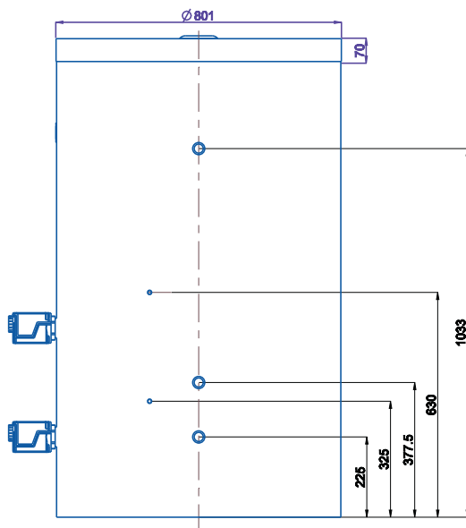
Aansluitingen afgiftesysteem
