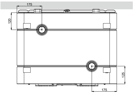
Onderaanzicht
