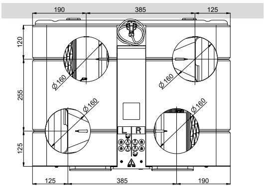
Bovenaanzicht
